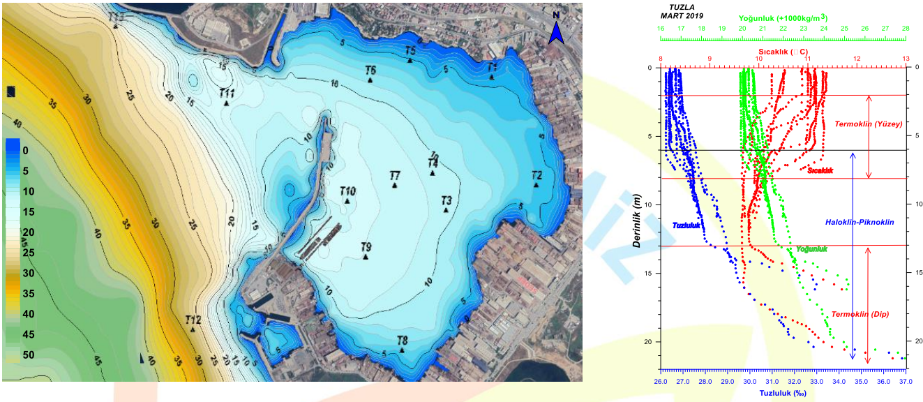
Tuzla Tersaneler Bölgesi Batimetri Haritası (Sol) ve Deniz Suyu Ortamsal Parametreleri (Sağ)
