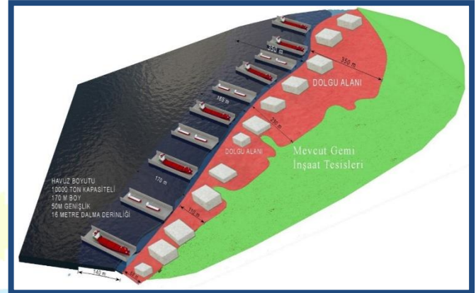
Aliağa Gemi Geri Dönüşüm Tesisleri Bölgesi'nde Yüzer Havuzlardan Yararlanma Seçeneği
